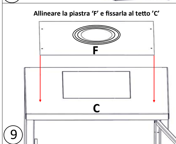
OPZIONE 'B': CHIUSURA PORTA DA SX VERSO DX
