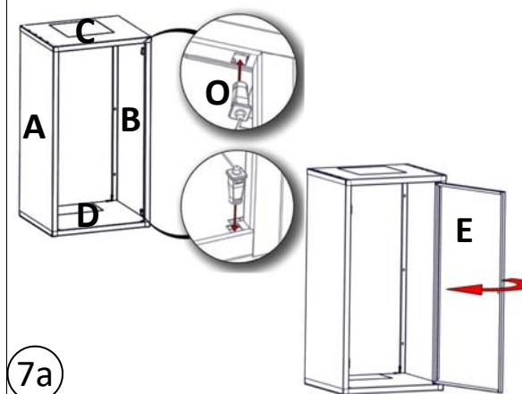
OPZIONE 'A': CHIUSURA PORTA DA DX VERSO SX
